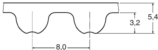
8M (nur Mittelwerte nominal dimensions – mm)
